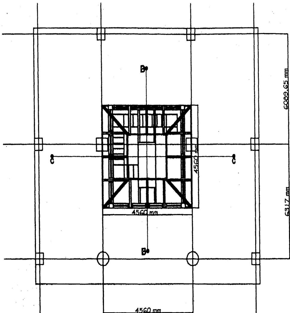
Top view Scale: 1:1
